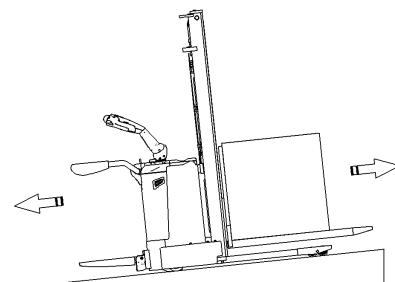
Рис..10: Движение по уклону
