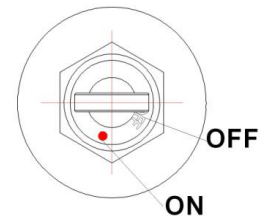
Рис.8: Замковый выключатель
