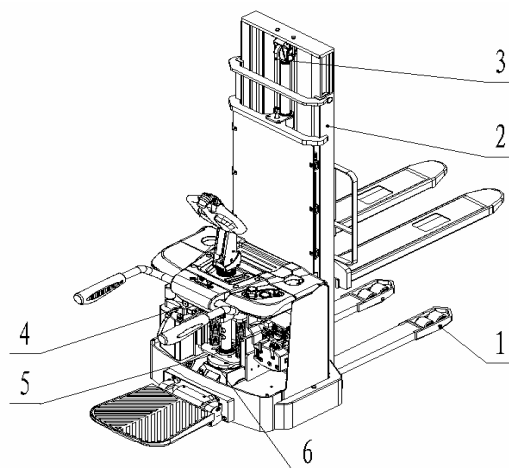
Рис.15: Места смазки
