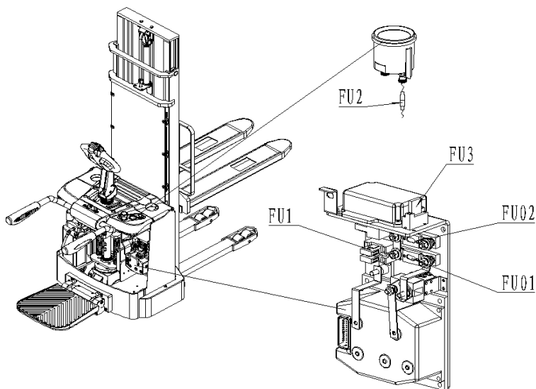
Рис. 16: Расположение предохранителей
